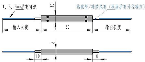
A. 方形铝盒型（无安装孔）
