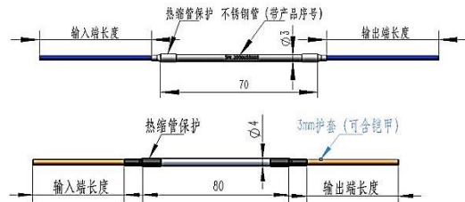
B. 不锈钢管型
